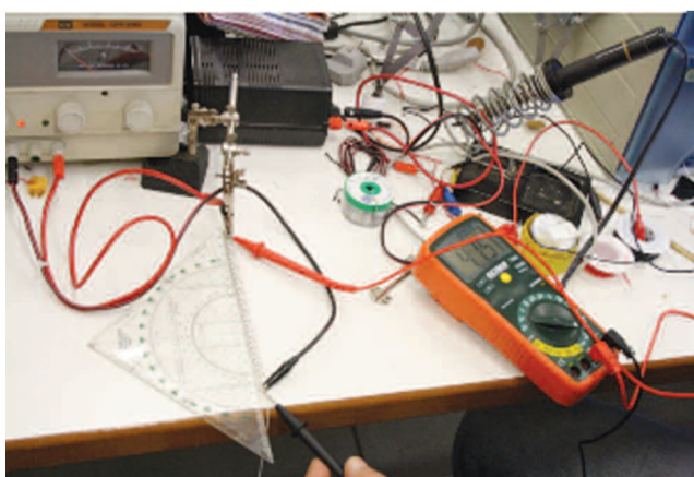
Πειράματα κίνησης του ελατηρίου Nitinol.
