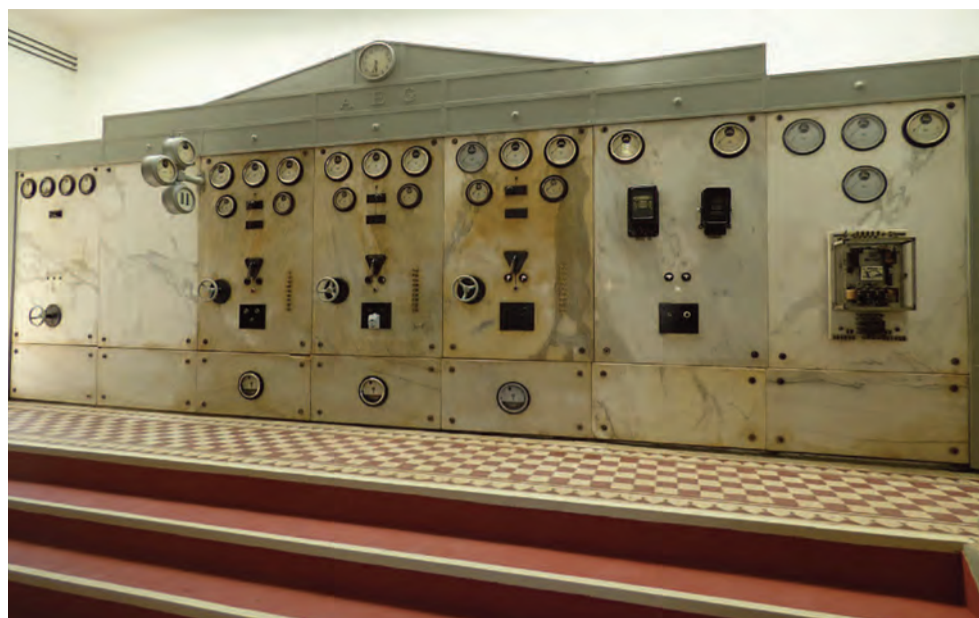
Ο μαρμάρινος πίνακας ελέγχου διασώζεται μέχρι σήμερα.
